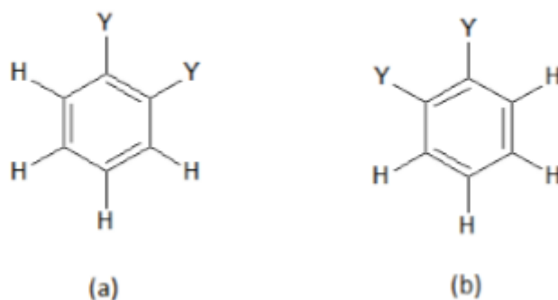
Slika 2.6.2.4. Orto-izomeri benzena
