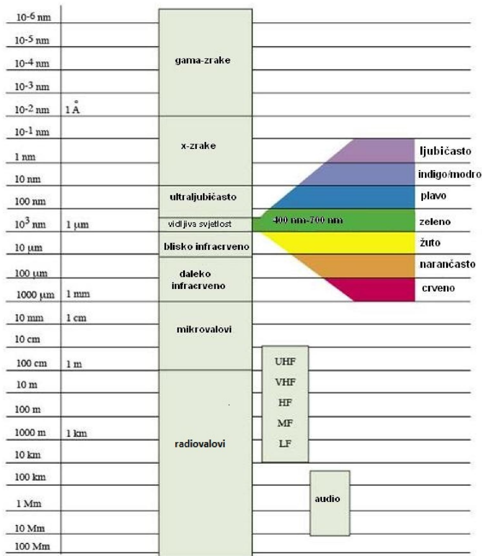
Slika 7. Elektromagnetski spektar
