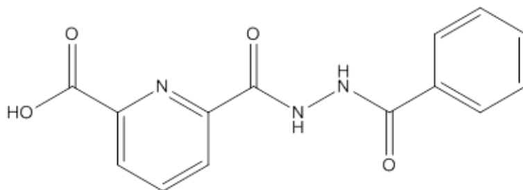
Slika 3. Prikaz strukture 6-(2-benzoylhidrazinyl)picolinske kiseline
