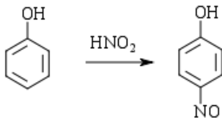
Slika 16. Nitroziranje fenola
