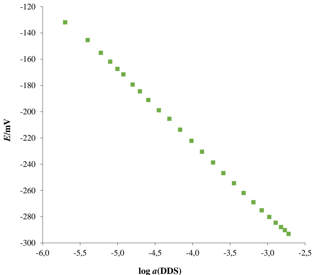
Slika 28. Odzivne karakteristike DDA-TPB senzora u otopini \text{Na}_2\text{SO}_4 koncentracije c = 1 \cdot 10^{-2} mol/L prema otopini NaDS-a.
