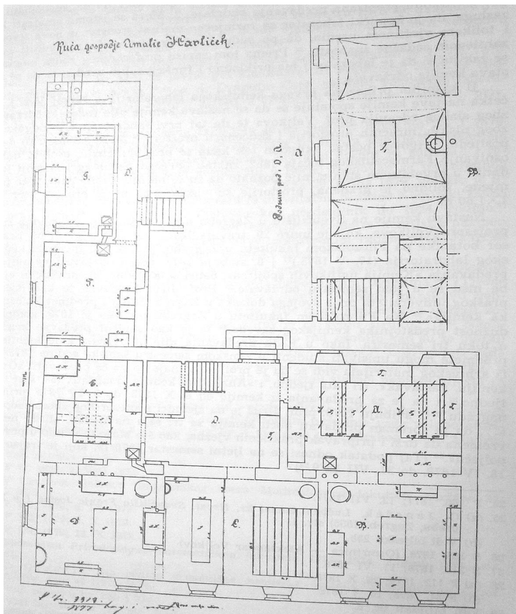
SLIKA 4. Tlocrt prvog kemijskog zavoda u Novoj Vesi br.1 iz 1877. Godine [3]
