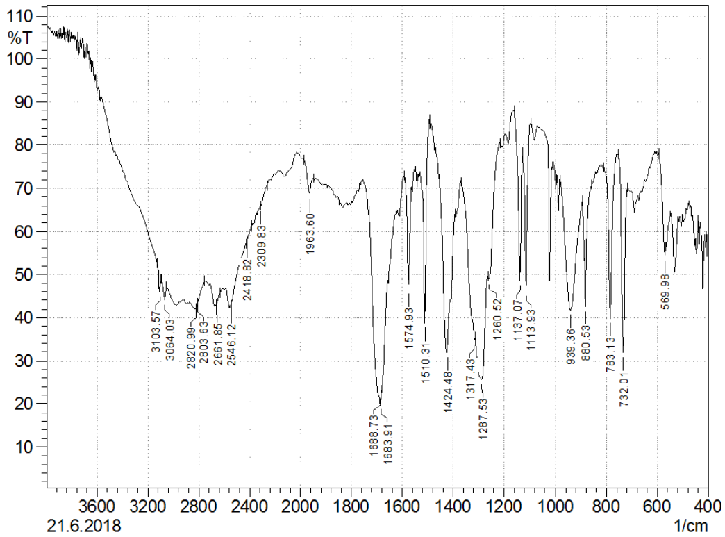
Slika 26. FeMOF-5aDV
