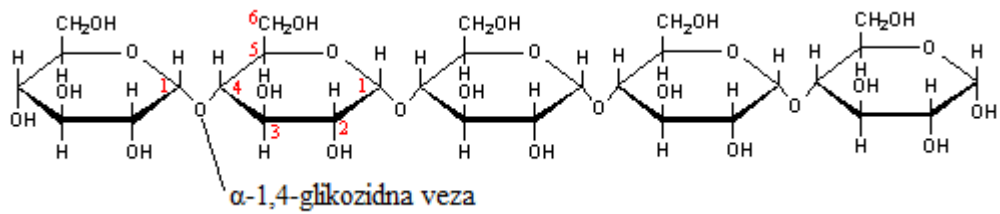
Slika 7: Amiloza
