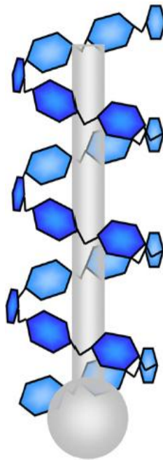
Slika 8: Kompleks amiloza-tenzid
