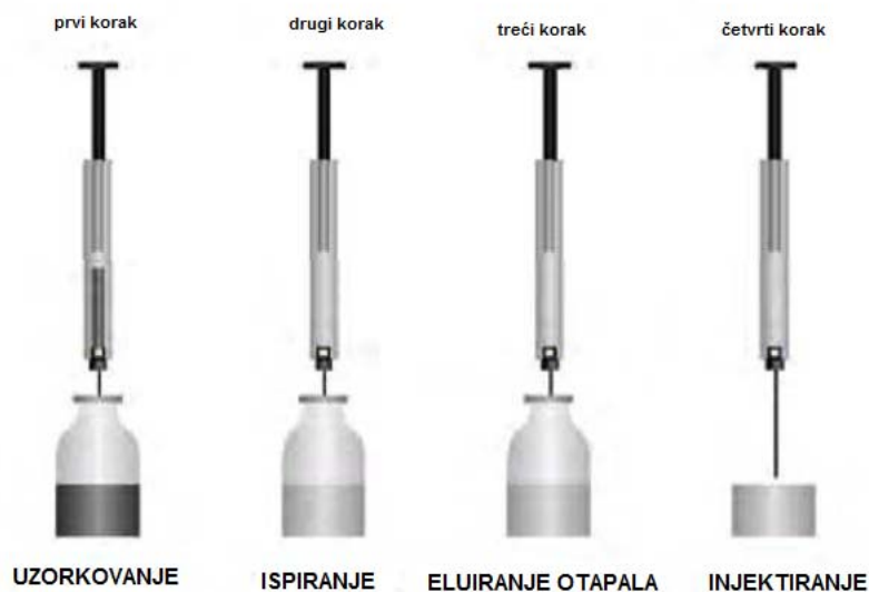
Slika 11. Koraci MEPS-a [49].
