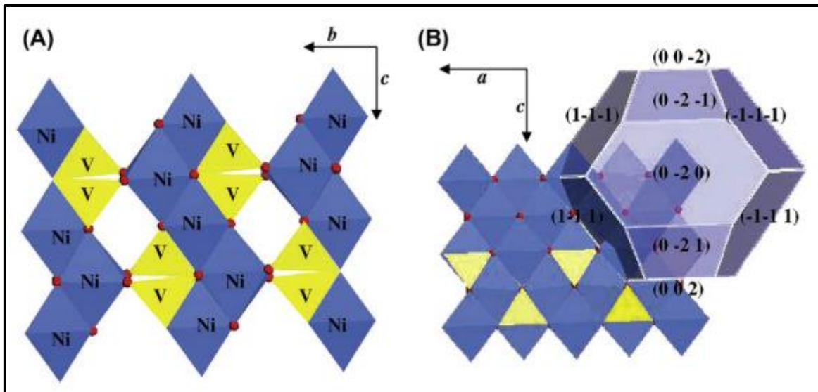
Slika 10. Projekcija kristalne strukture Ni_3V_2O_8 na (A) b - c ravninu i (B) a - c ravninu [5].
