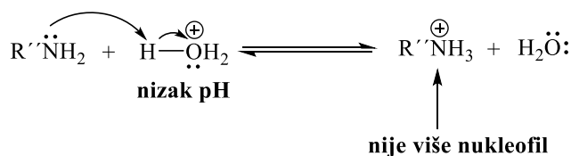
Slika 8. Protoniranje amina jakom kiselinom [4].
