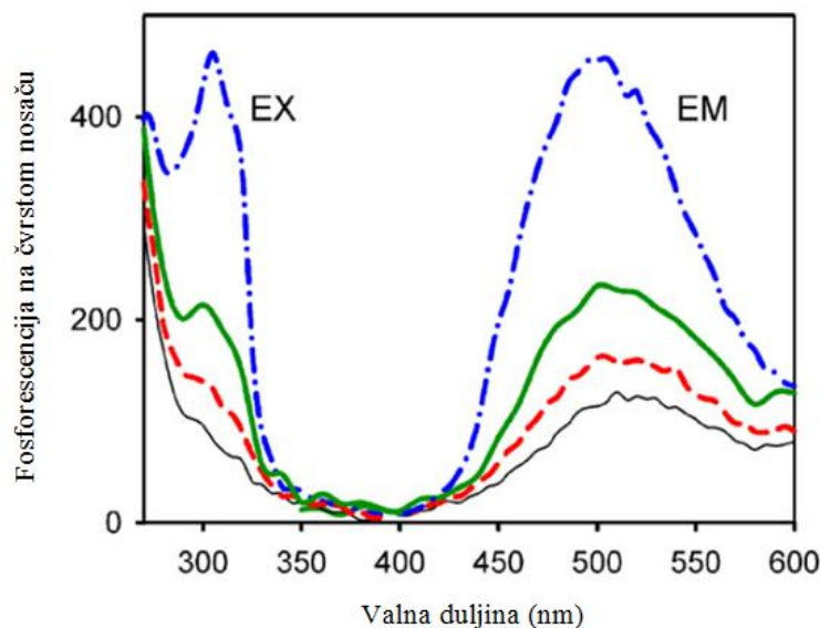
Slika 11. Ekscitacijski (EX) i emisijski (EM) spektar fosforescencije tiabendazola imobiliziranog na najlonu (crvena isprekidana linija), u prisutnosti KI (zelena linija) te u prisutnosti KI i \text{Na}_2\text{SO}_3 (crna linija su pozadinski signali) [43].
