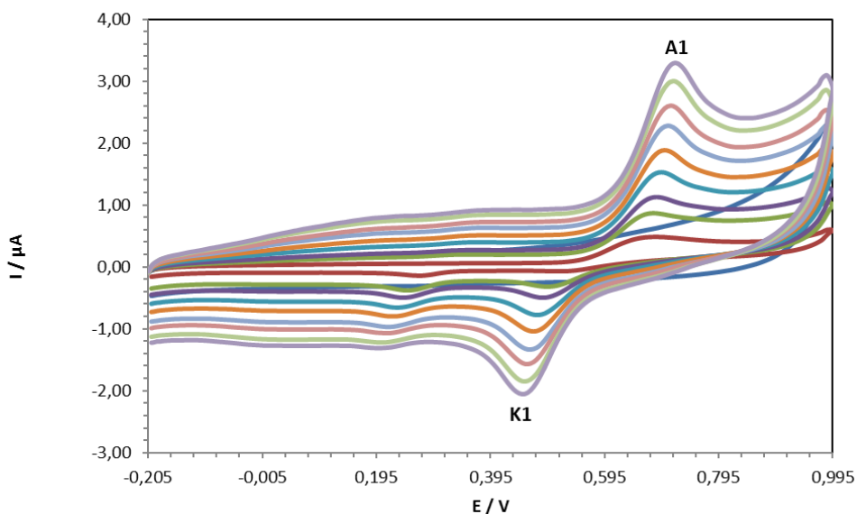
Slika 12. Ciklički voltamogrami Zn_3L_3 kompleksa snimljeni na elektrodi od staklastog ugljika u KCl inertnom elektrolitu ( c = 0,1 \text{ M} ) pri različitim brzinama polarizacije elektrode, v = 20\text{-}400 \text{ mV/s} .
