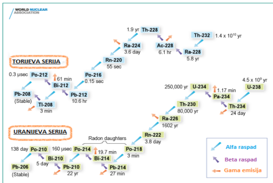
Slika 1. Shematski prikaz torijeva i uranijeva lančane serije radioaktivnog raspada. [13]
