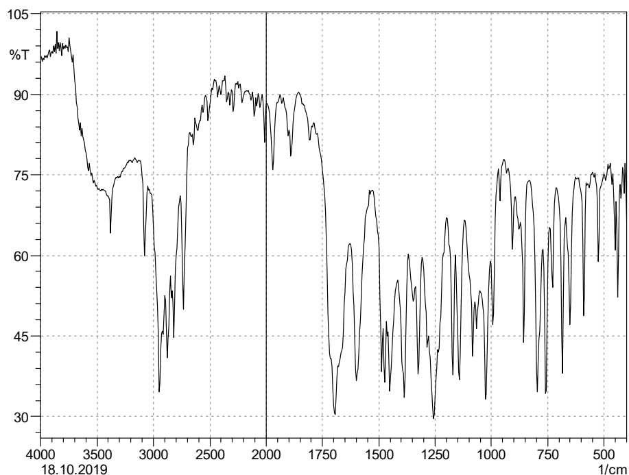
Slika 19. FTIR spoja 2
