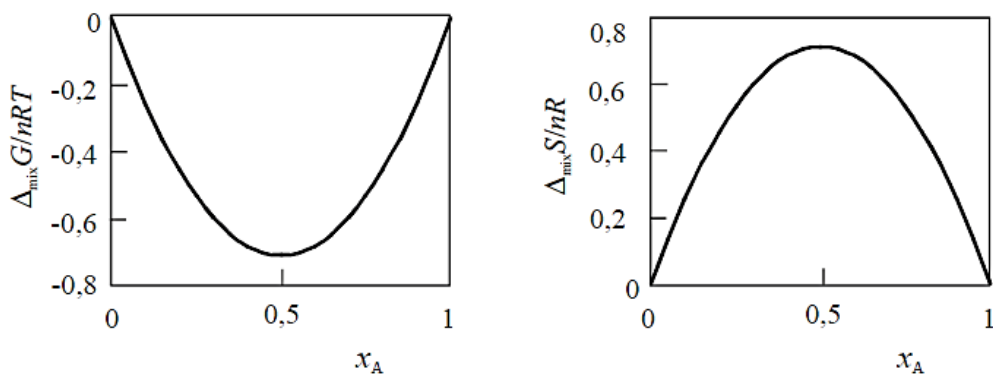
Slika 2. Prikazana je ovisnost Gibbsove energije ( \Delta_{\text{mix}}G ) i entropije ( \Delta_{\text{mix}}S ) miješanja dvaju idealnih plinova pri stalnom tlaku i temperaturi o sastavu nastale smjese [6].
