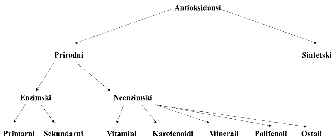
Slika 7. Podjela antioksidansa [52].
