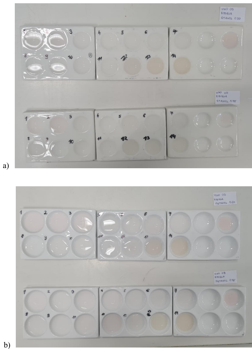
Slika 88. Vino od crvenog ribiza s dodanim a) etanolom (50 %, gore i 75 %, dolje) i b) metanolom (50 %, gore i 75 %, dolje).
