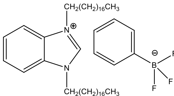
Slika 21. Strukturna formula 1,3-dioktadecil-1 H -benz[ d ]imidazol-3-ijeve trifluoro(fenil)borata (4).
