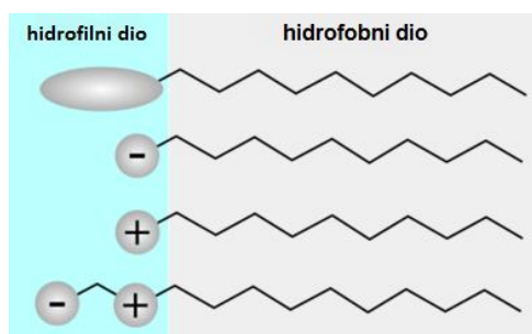
Slika 3: Shematski prikaz molekule tenzida
