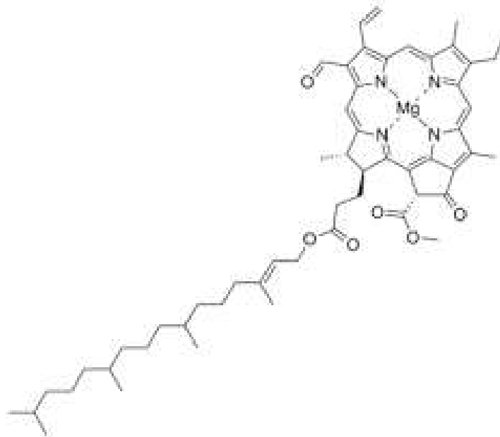
Slika 20. Struktura klorofila [48].
