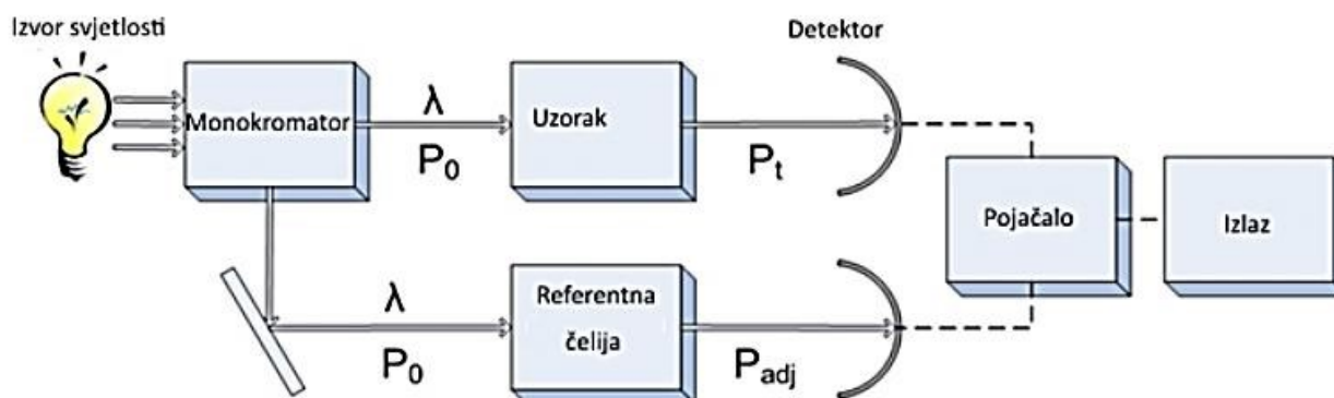
Slika 9. Shematski prikaz dvosnopnog smektrofotometra [27].
