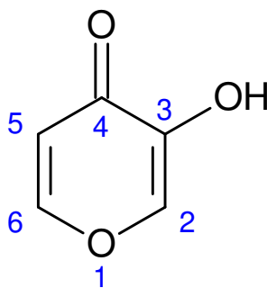
Slika 2. Opća strukturalna formula 3-hidropsipiran-4-on.
