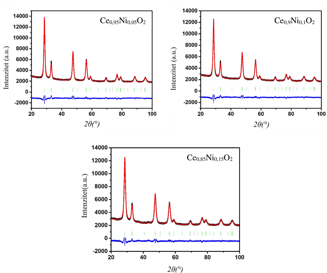
Slika 17. Difraktogrami \text{CeO}_2 dopiranih s 5 %, 10 % i 15 % Ni
