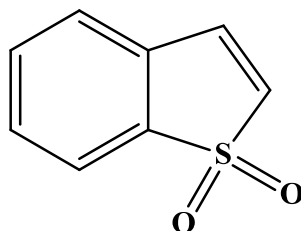
Slika 19. Kemijska struktura benzo[ b ]tiofen 1,1-dioksida (3)
