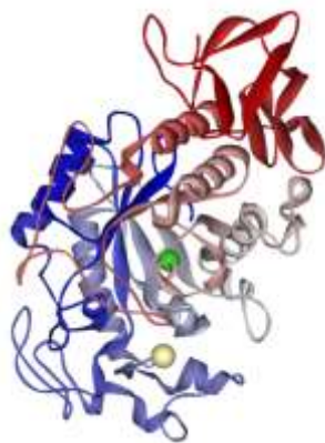
Slika 4. Shematski prikaz strukture \alpha -amilaze iz sline s kalcijevim ionom u aktivnom centru (zeleno kuglica predstavlja kalcij)[14]
