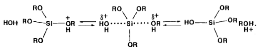
Slika 2.4. Mehanizam kiselo-katalizirane hidrolize tetraalkoksisilana [14].
