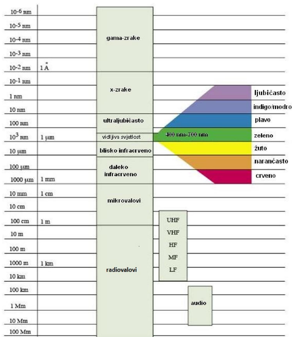
Slika 7. Elektromagnetski spektar
