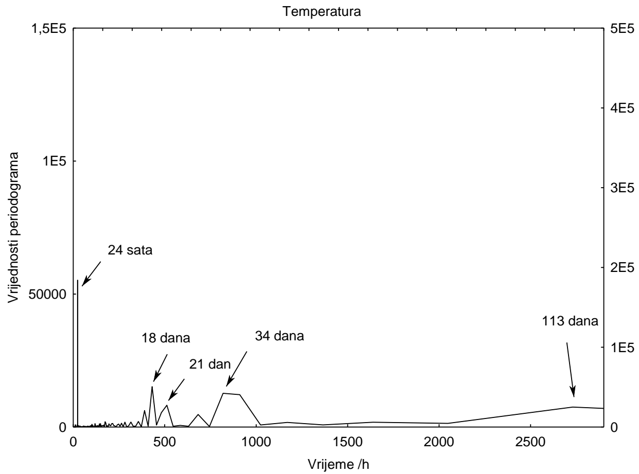
Slika 14. Fourierov spektar temperature, prikaz kraćeg vremenskog perioda
