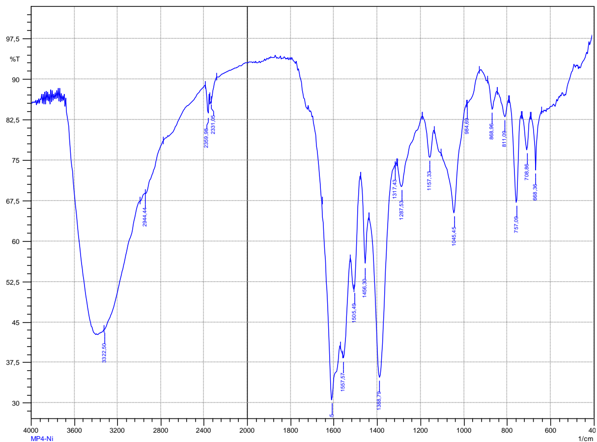
Slika 7. IR spektar kompleksa (ksi-antr) 2 Ni
