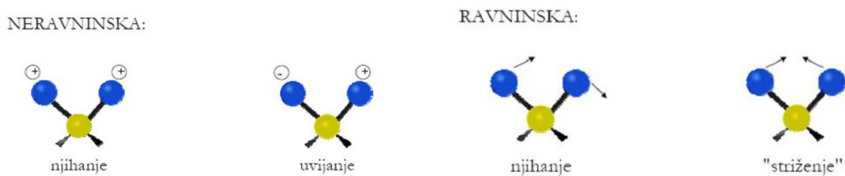
Slika 2. Neravninska i ravninska deformacija kuteva
