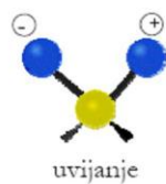
Slika 2. Neravninska i ravninska deformacija kuteva
