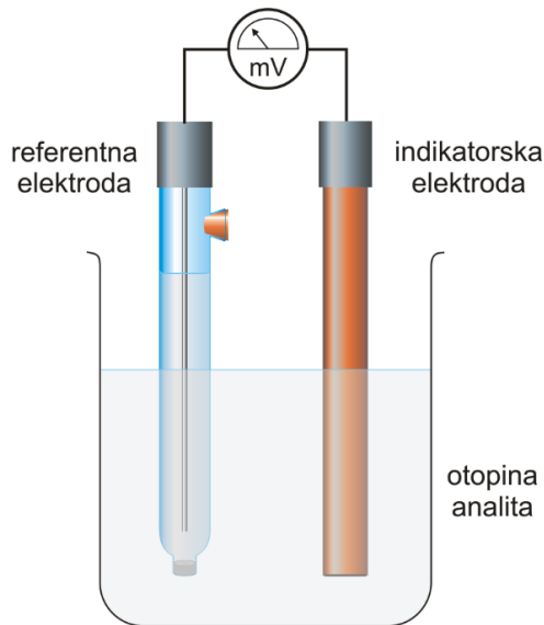
Slika 2.19. Elektrokemijska ćelija za potenciometrijsko mjerenje [27].
