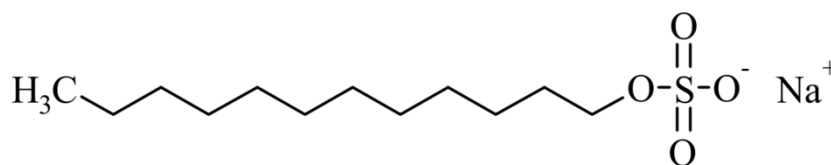
Slika 19. Strukturna formula natrijeva dodecilsulfata.
