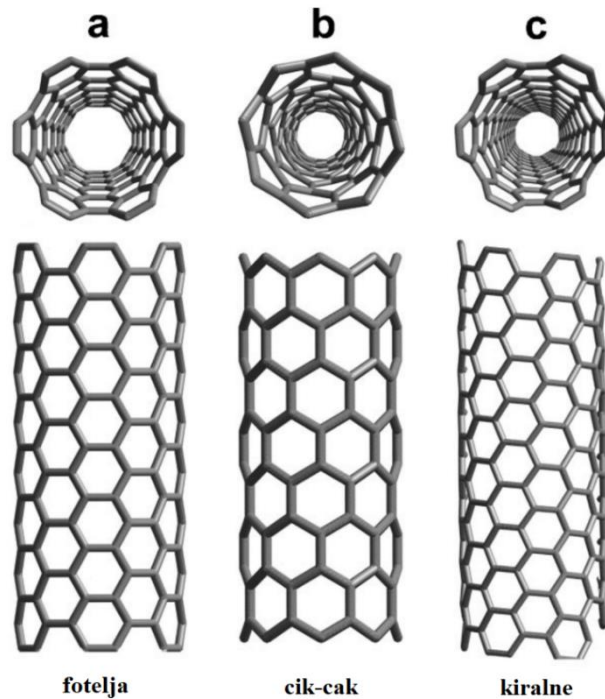
Slika 17. Tipovi nanocjevčica [49].
