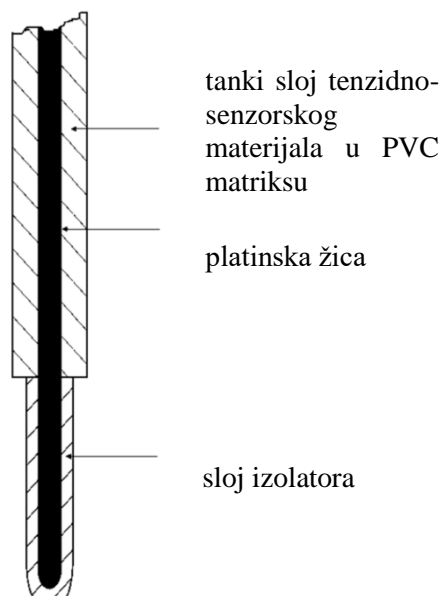
Slika 15. Shema ion-selektivne coated-wire elektrode [45].
