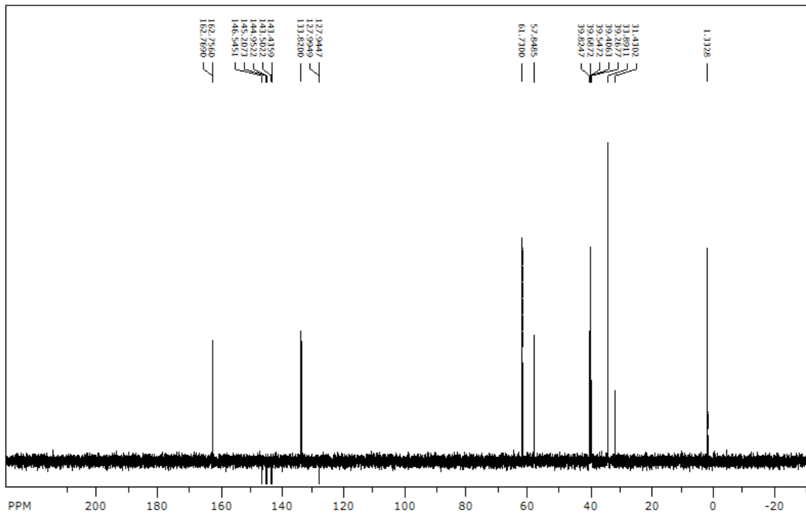
Slika 30. 13 C spektr 3-karbamoil-1-(3-jodopropil)-piridinijeva jodida (3)
