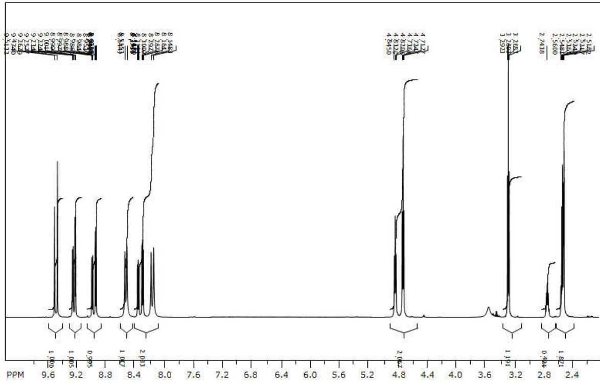
Slika 29. 1 H spektr 3-karbamoil-1-(3-jodopropil)-piridinijeva jodida (3)
