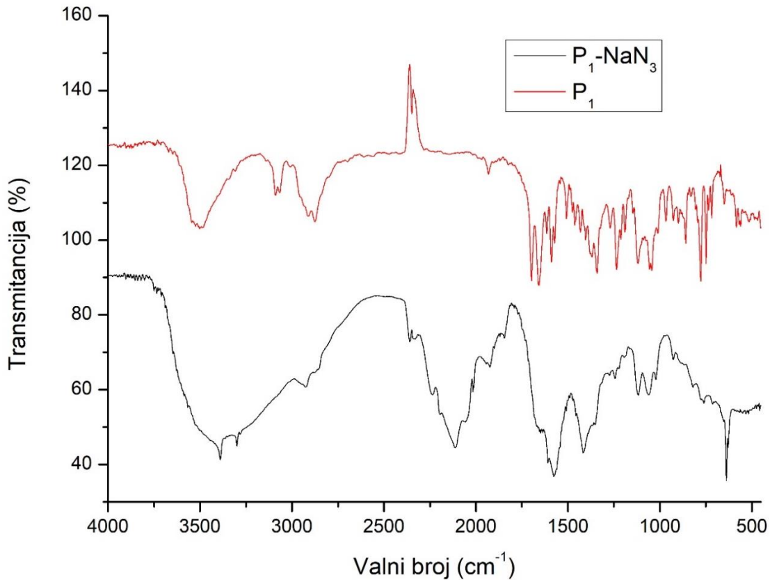
Slika 28. Usporedba FT-IR spektara P_1 -NaN 3 i P_1
