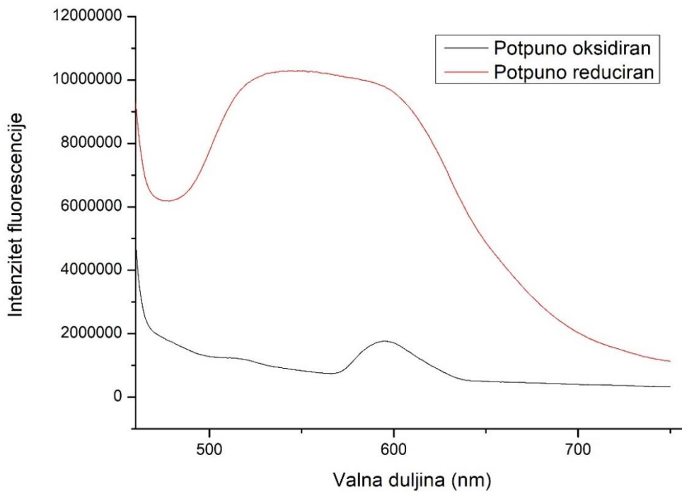
Slika 32. Usporedba intenziteta fluorescencije potpuno oksidiranog i potpuno reduciranog oblika Se-P 1
