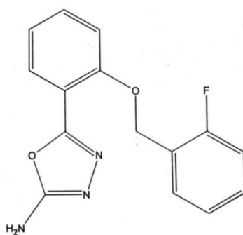
Slika 13. 5-{2-[(2-fluorobenzil)oksi]fenil}-1,3,4-oksadiazol-2-amin [13].
