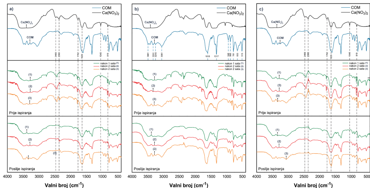
Slika 7 – IR spektri sintetiziranih uzoraka pri brzinama od a) 250 o/min, b) 500 o/min i c) 750 o/min uspoređenih s IR spektrom COM standarda i reaktanta \text{Ca}(\text{NO}_3)_2
