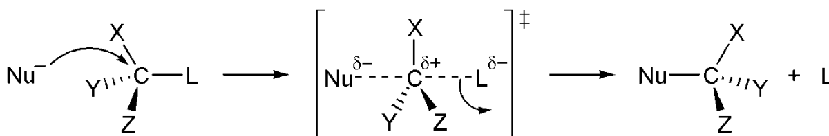
Slika 11. S_N2 mehanizam
