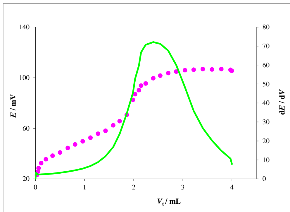
Slika 21. Potenciometrijska titrationska krivulja (●) i njena prva derivacija (—) za NaDDS ( c = 4 \cdot 10^{-3} mol/L) uz CPC ( c = 4 \cdot 10^{-3} mol/L) kao titrant i DDA-TPB_C senzor kao detektor završne točke titracije.
