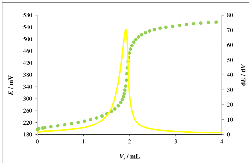
Slika 20. Potenciometrijska titrationska krivulja (●) i njena prva derivacija (—) za NaDDS ( c = 4 \cdot 10^{-3} mol/L) uz CPC ( c = 4 \cdot 10^{-3} mol/L) kao titrant i DDA-TPB_B senzor kao detektor završne točke titracije.
