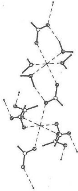
Slika 12. Prikaz vezanja kristalne strukture kobaltovogformijata (tamne kugle- atomi kobalta, svijetle kugle- atomi kisika). [10]
