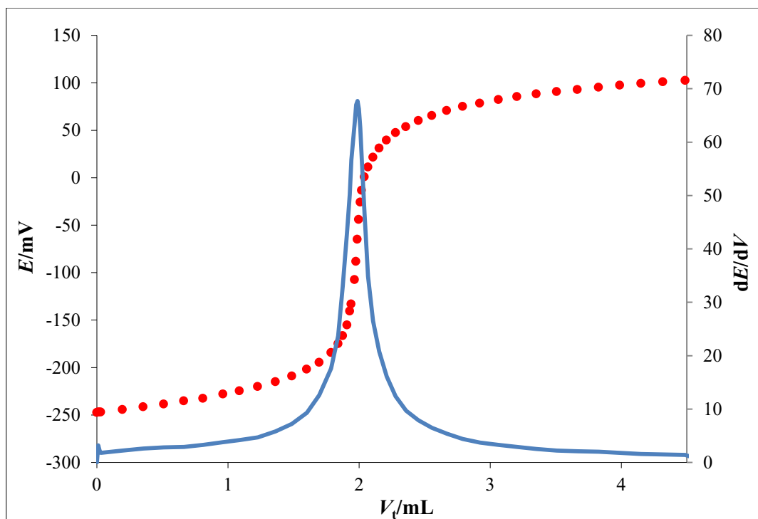
Slika 27. Potenciometrijska titracijska krivulja (●) i njena prva derivacija (—) za NaDDS ( c = 4 \cdot 10^{-3} \text{ mol dm}^{-3} ) uz CPC ( c = 4 \cdot 10^{-3} \text{ mol dm}^{-3} ) kao titrans i MJ1-TPB senzor kao detektor završne točke titracije
