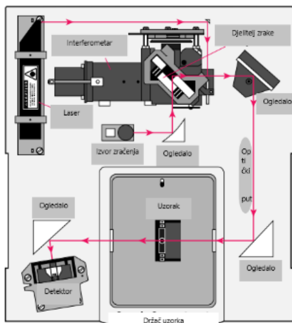
Slika 8. Shematski prikaz FT-IR spektrometra [63].
