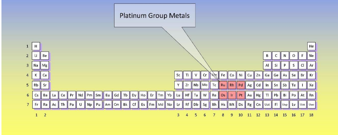
Slika 1. Položaj platinskih metala u periodnom sustavu elemenata. [12]
