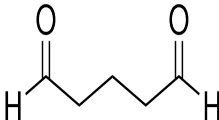
Slika 9. Glutaraldehyd [18]
