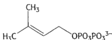
Slika 5.: Dimetilalil-pirofosfat [2]
