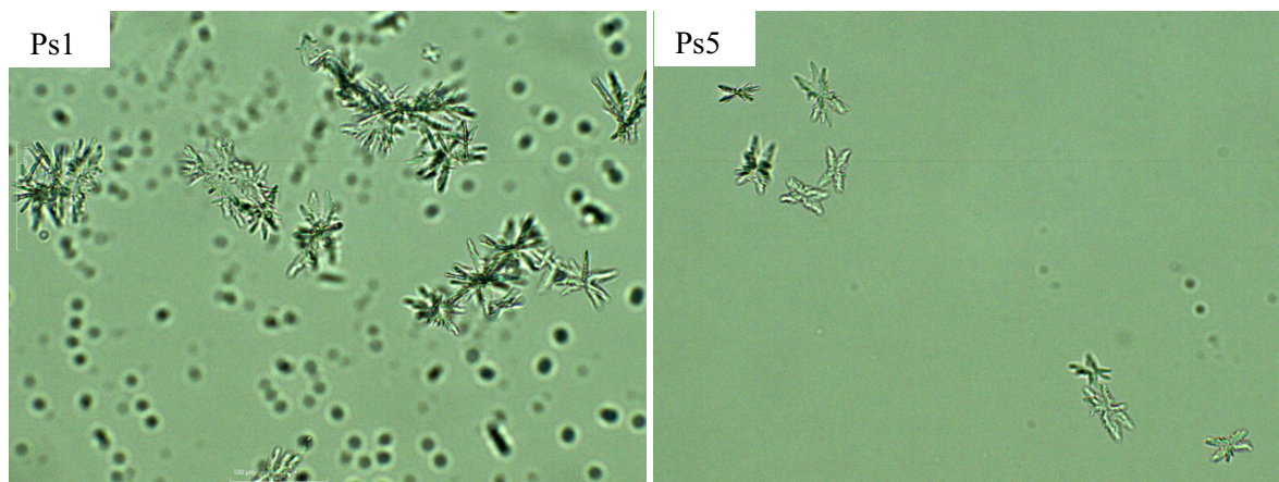
Slika 17. Morfologija kristala kalcijeva oksalata u sustavu Ps1 i Ps5.
