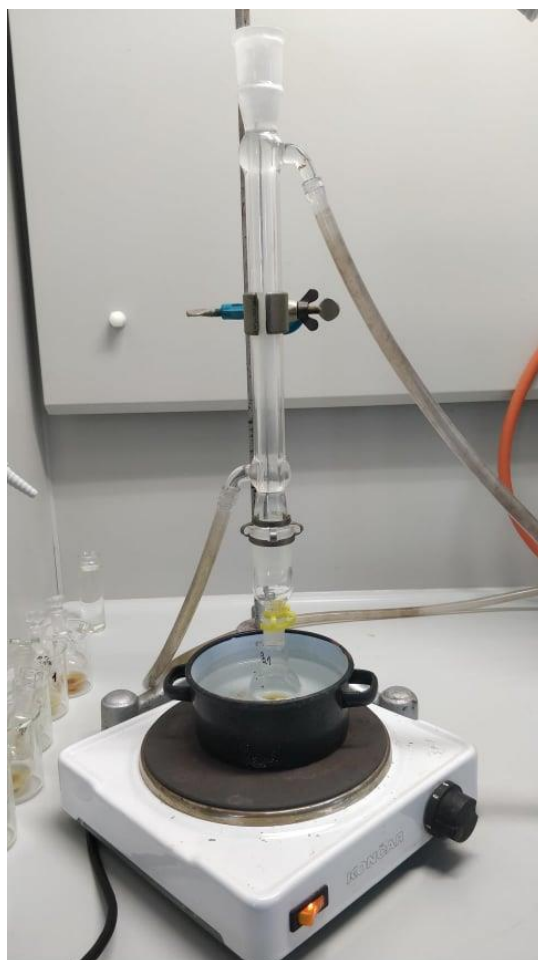
Slika 40. Aparatura za hidrolizu i esterifikaciju
