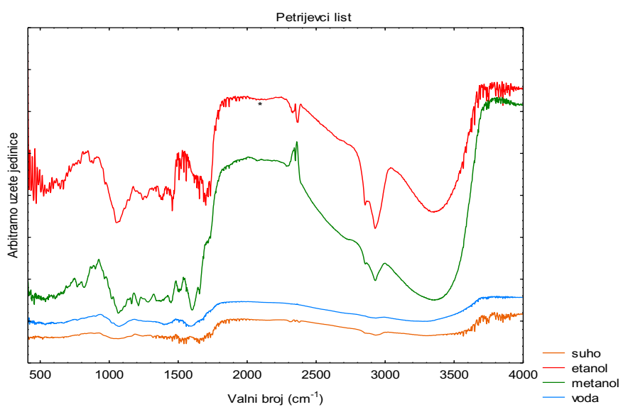
Slika 16. FTIR spektri listova imele s područja Petrijevac (etanol, metanol i voda u usporedbi sa suhim uzorkom)
