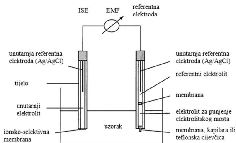
Slika 11. Shema potencijometrijskog sustava za mjerenje.
