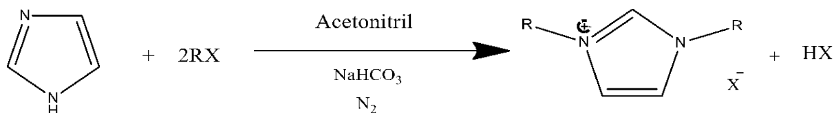
Slika 34. Jednadžba kemijske reakcije kvaternizacije ( R=18 , X=\text{bromid} )
