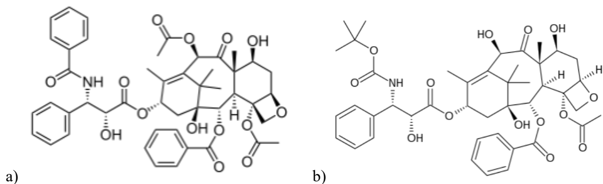
Slika 11. Struktura a) paklitaksela [45] i b) docetaksela [46].
