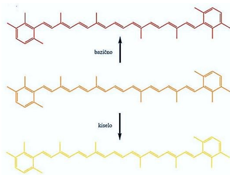
Slika 7. Struktura i boja karotenoida u bazičnom (gore), neutralnom (sredina) i kiselom (dolje) mediju [37].
