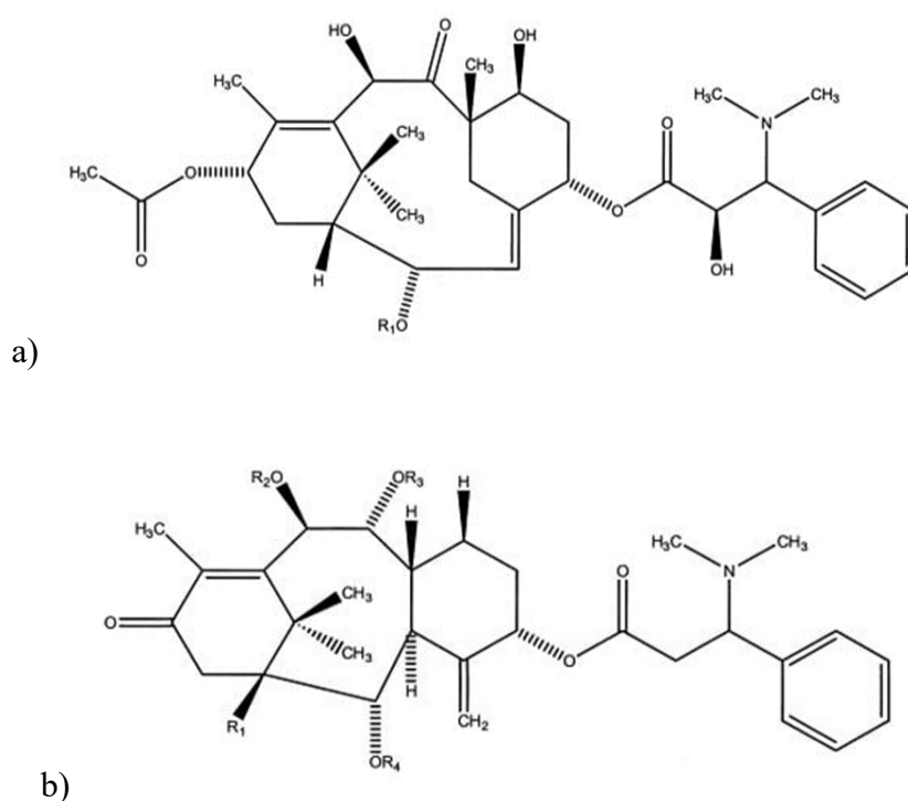
Slika 10. Struktura a) taksina A i b) taksina B [43].
